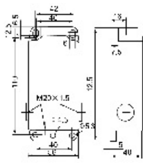
LXP1-404壳体尺寸
